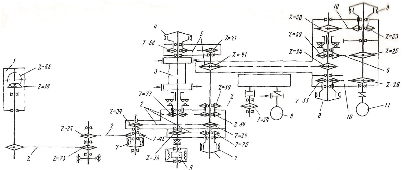
Рисунок 1 – Кинематическая схема привода лебедки и ротора БУ-3000ЭУК 1-ротор; 2,5,10-соответственно двухрядная, трехрядная и четырехрядная роliko-втулочные цепи t=50,8 ; 3- лебедка; 4,7,9- шинно-пневматические муфты диаметрами 1070, 500 и 700мм; 8- регулятор подачи долота РПД; 11- электродвигатель привода лебедки
