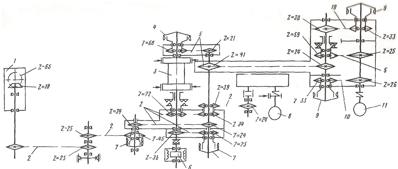
Рисунок 1 – Кинематическая схема привода лебедки и ротора БУ-3000ЭУК
