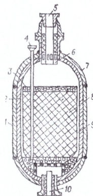
Рисунок 1- Реактор риформинга с аксиальным вводом газо-сырьевой смеси:
